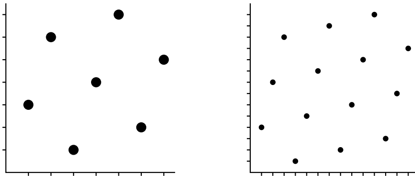
Figure 3: \pi^{(4)} = 3\ 6\ 1\ 4\ 7\ 2\ 5 , and \pi^{(5)} = 4\ 8\ 12\ 1\ 5\ 9\ 13\ 2\ 6\ 10\ 14\ 3\ 7\ 11
